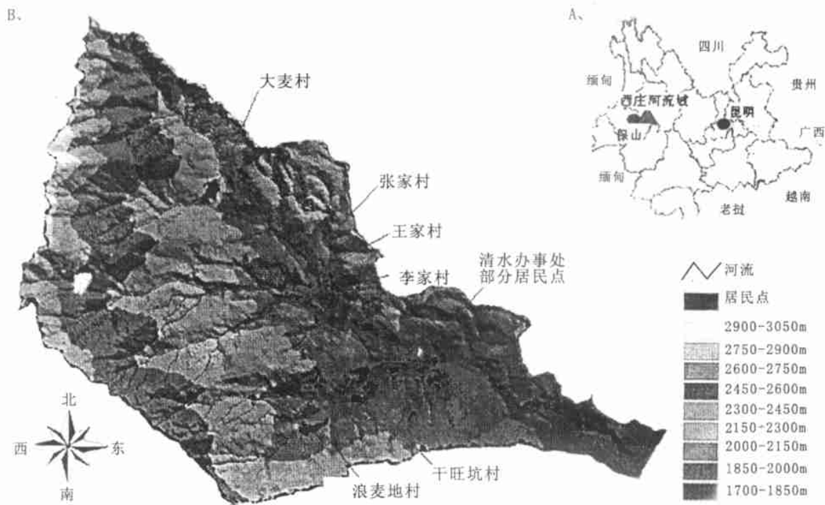
图 1 西庄河山地流域位置图及流域轮廓图(a 西庄河流域位置图; b 流域轮廓图及居民点分布略图)
