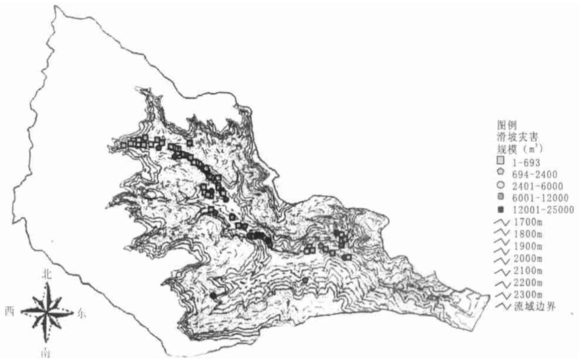
图 2 滑坡灾害调查区域及滑坡空间分布
