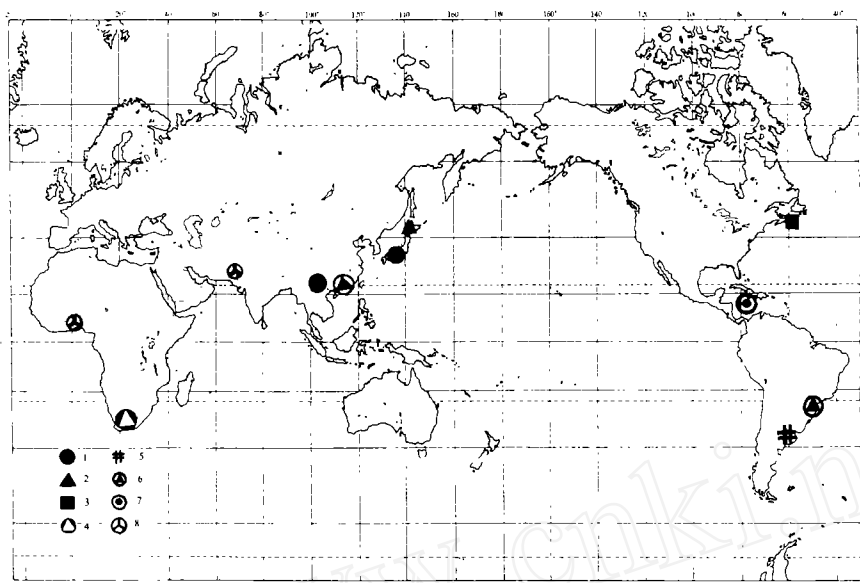
图2 原块菌属分布图
