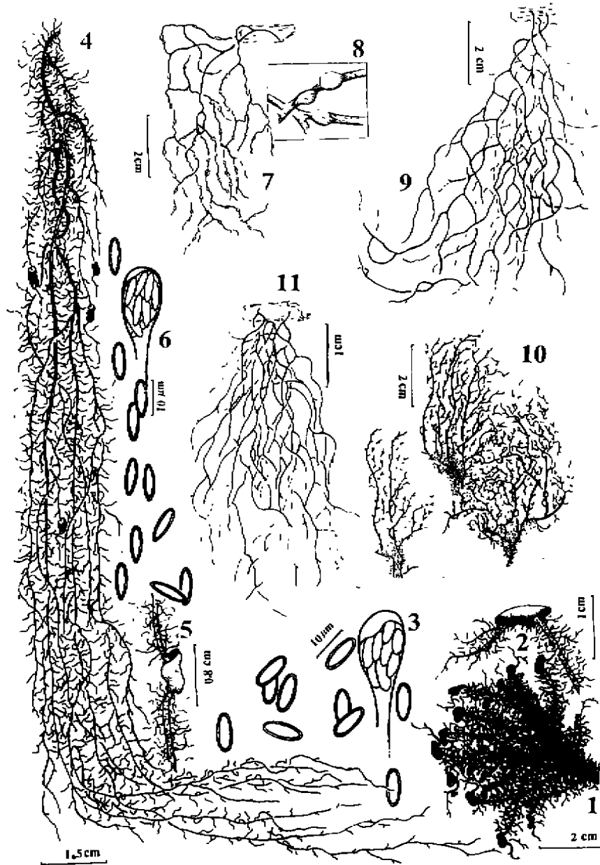
图 1 1. 广开小孢发 Bryoria divergescens , 2. 子囊盘及枝体局部放大; 3. 子囊及子囊孢子; 4. 喜马拉雅小孢发 B. himalayana ; 5. 子囊盘及枝体局部放大, 6. 子囊及子囊孢子; 7. 波氏小孢发 B. poeltii ; 8. 粉芽堆放大; 9. 光滑小孢发 B. levis ; 10. 光亮小孢发 B. nitidula , 11. 尼泊尔小孢发 B. nepalensis .
