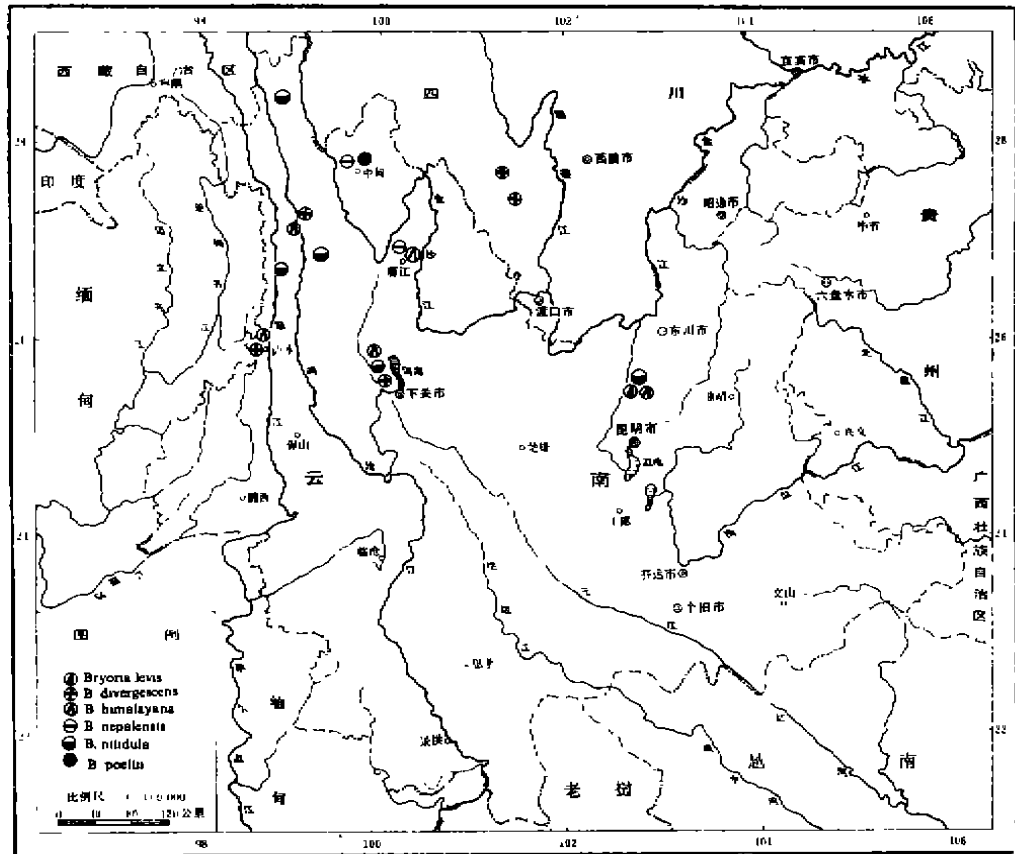
图 2 6 种云南小孢发属地衣的分布
