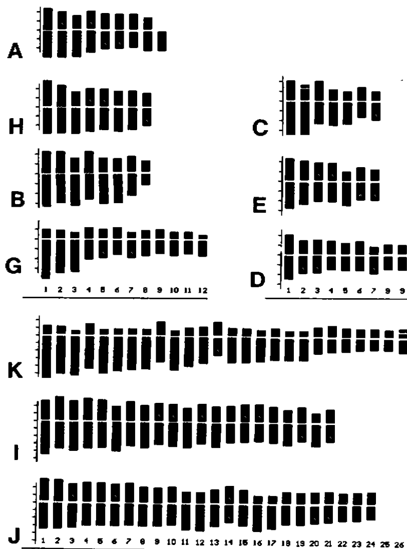
图 1 核型模式图
