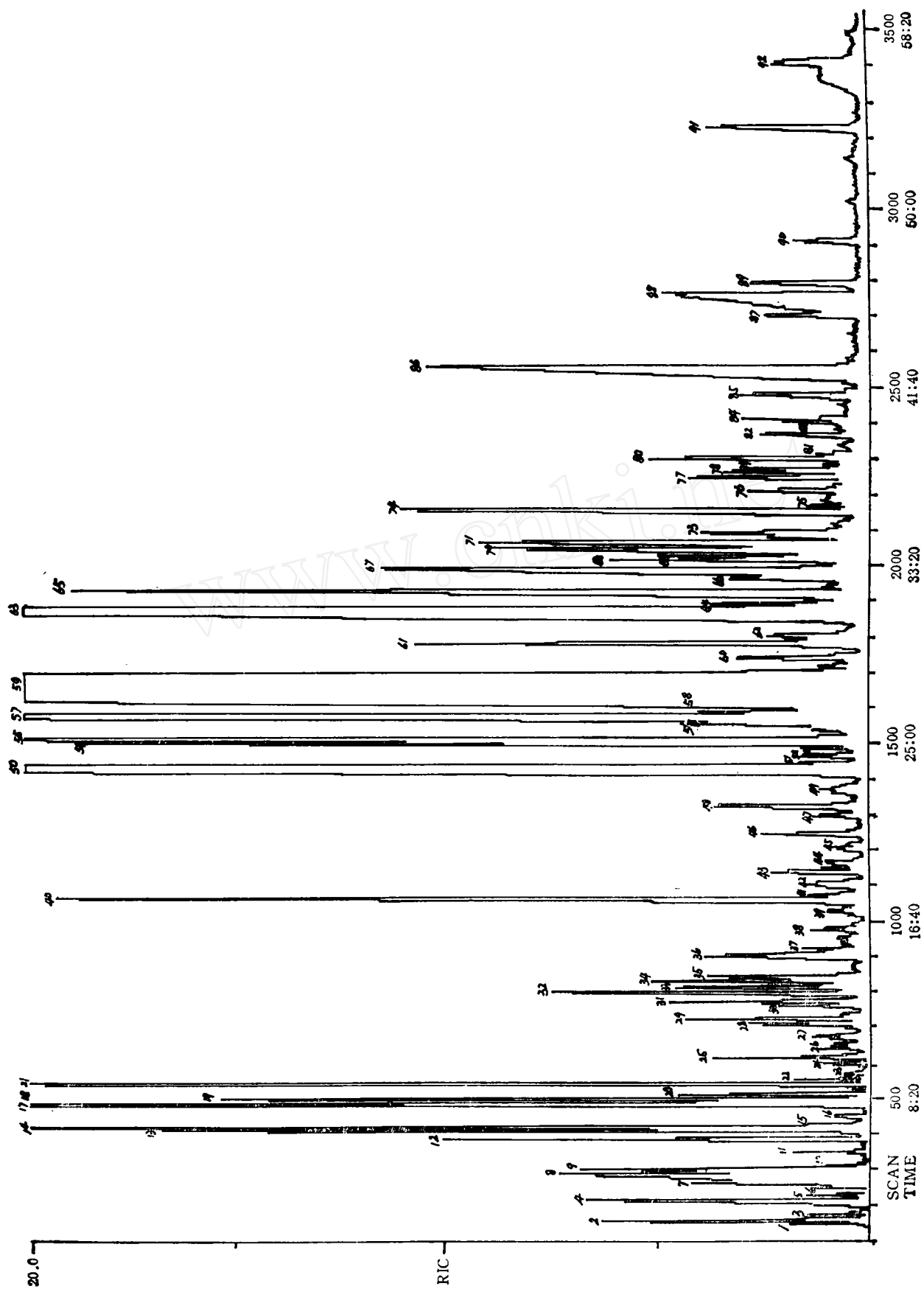
图1 猪毛蒿精油的气相色谱图
