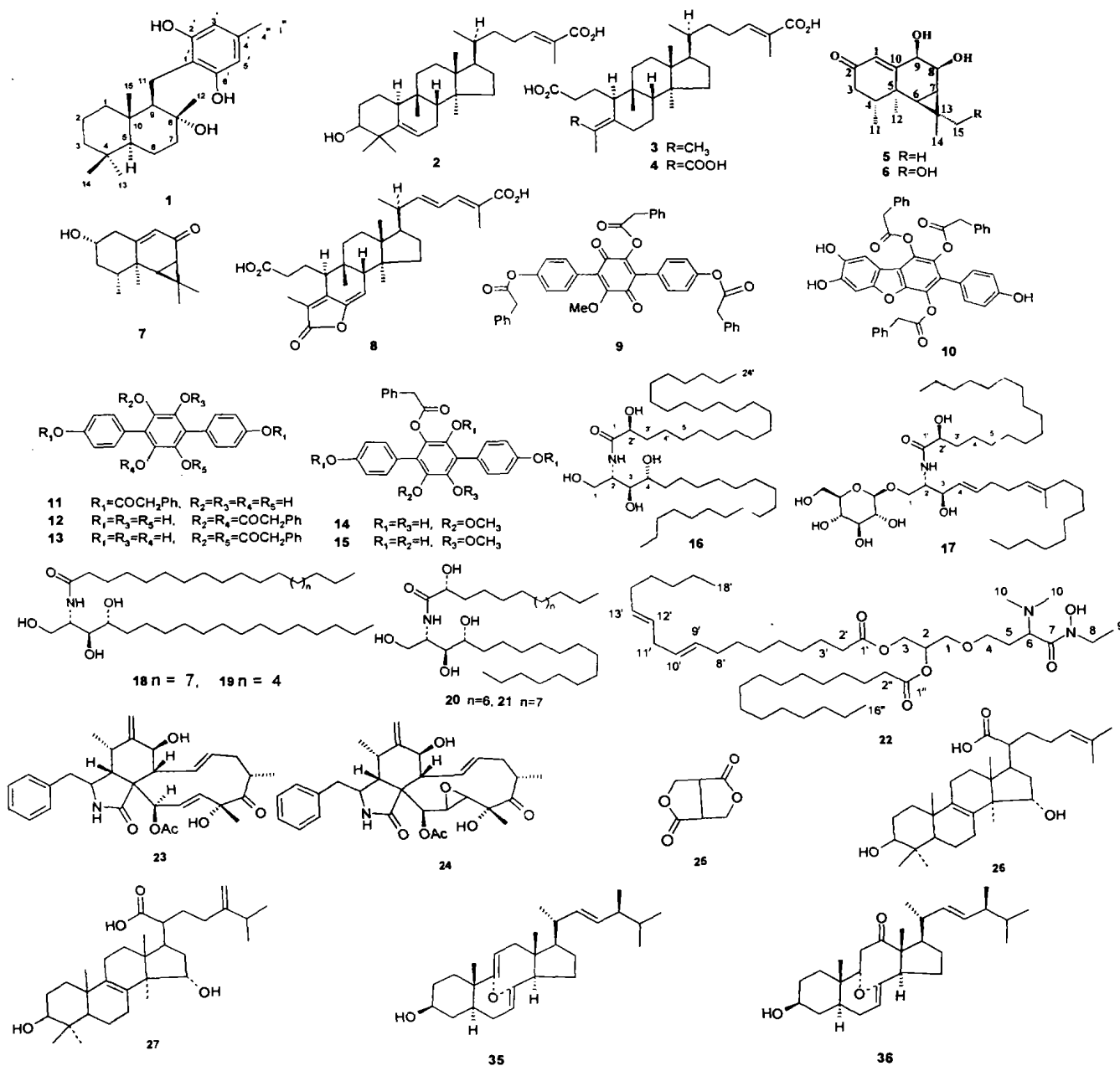
图 1 化合物 1~27, 35, 36 的化学结构
