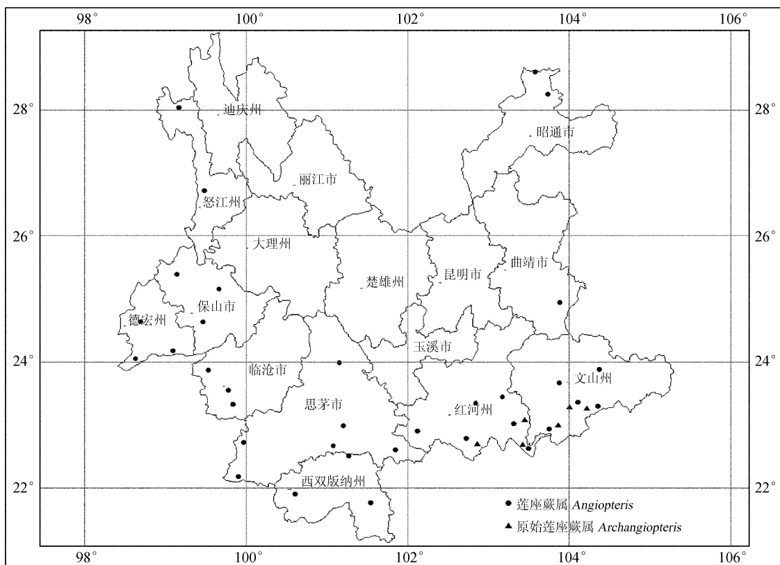
图 1 云南莲座蕨科植物分布示意图
