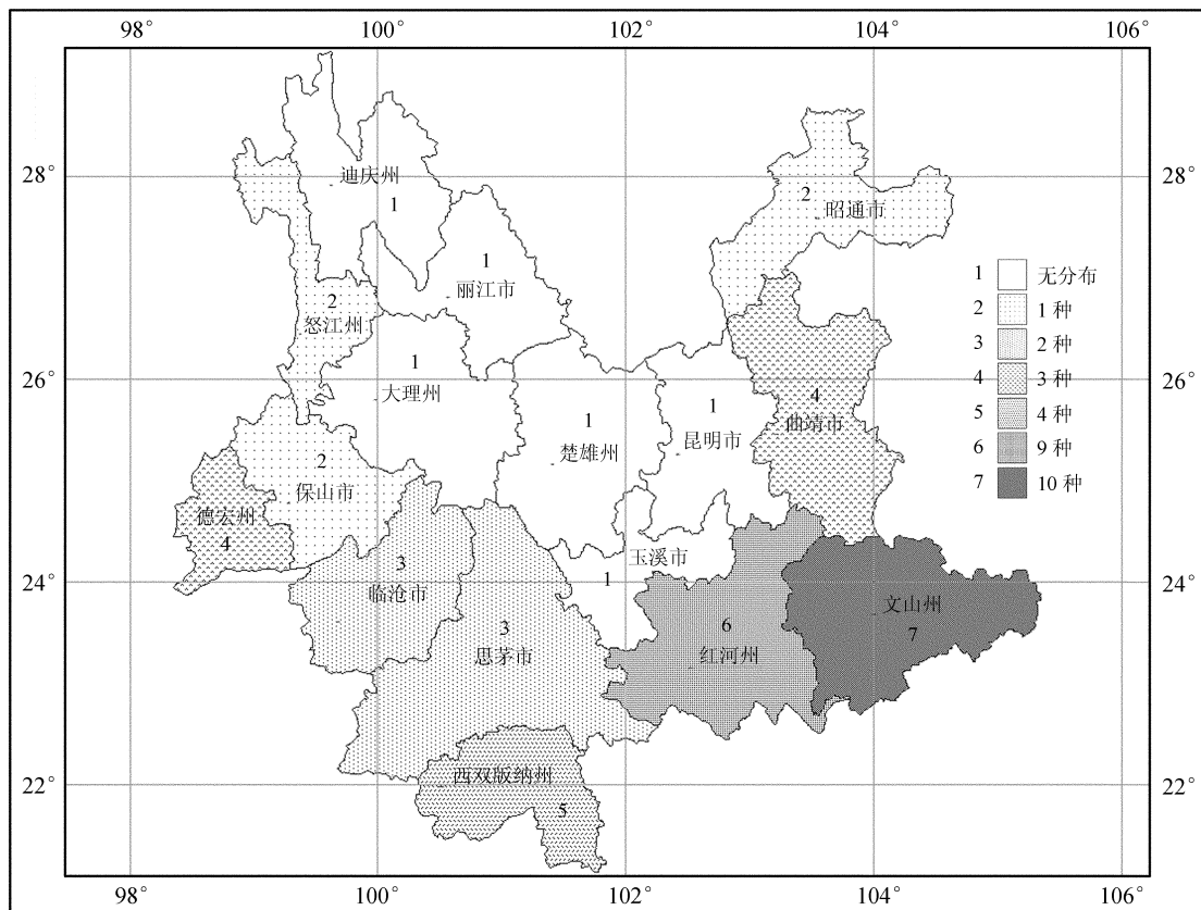
图 2 云南莲座蕨科物种分布丰富度图
