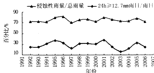
图3 侵蚀性雨量/总降雨量、 24 h \geq 12.7 mm 雨日/雨日的百分比年变化
