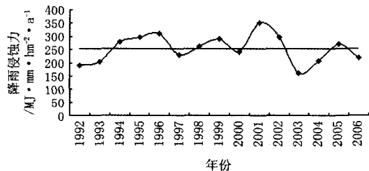
图 6 勐仑降雨侵蚀力年变化曲线(1992~2006 年)
