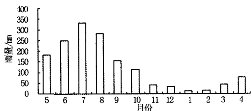
图2 1992~2006 期间降雨年内分配情况(水文年)
