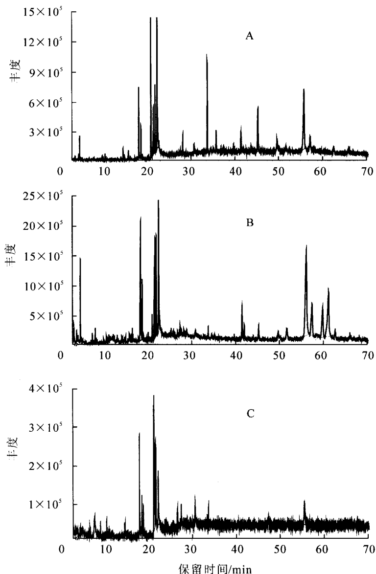
图 1 麻疯树叶(A)、树皮(B)和种子(C)乙醇加热回流提取物 GC-MS 总离子流图
