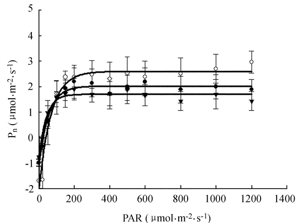
图 1 不同温度下铁皮石斛 (T-20 ●-●; T-30 ○-○; T-40 - ) 的光合作用对光照强度的响应, 误差条表示 3 次测量的标准误
