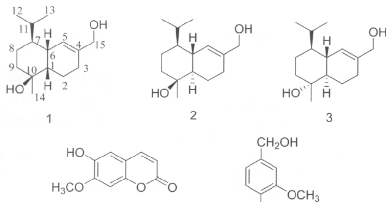
图 1 化合物 1—5 结构式
