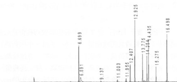
图 1 12 种有机磷农药混合对照图谱
