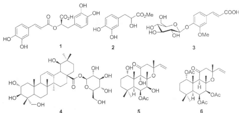
图 1 化合物 1-6 的结构式
