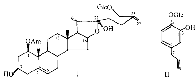
图 1 化合物 I 和 II 的化学结构式
