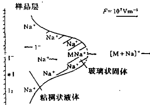
图1 FD-MS的离子化机制
