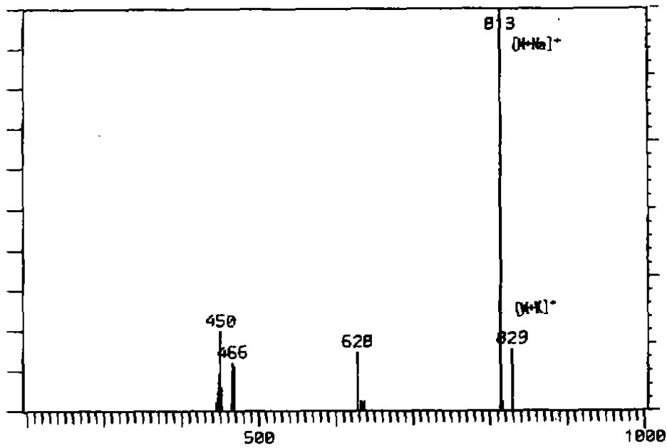
图 9 滇木犀榄甙(20)的 FD-MS 谱图
