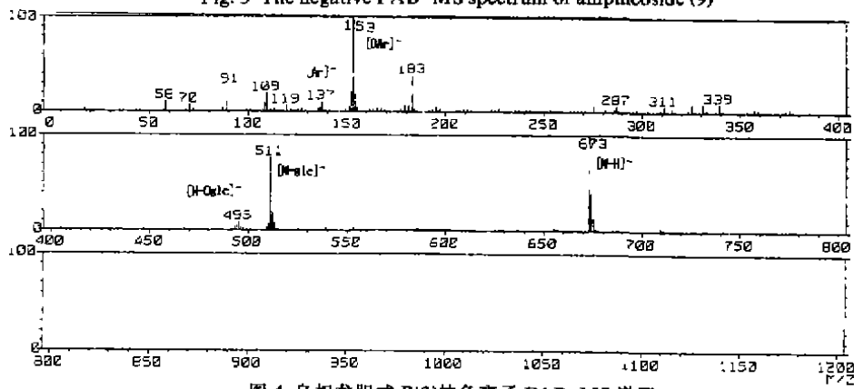
图4 乌奴龙胆甙 B(3)的负离子 FAB-MS 谱图
