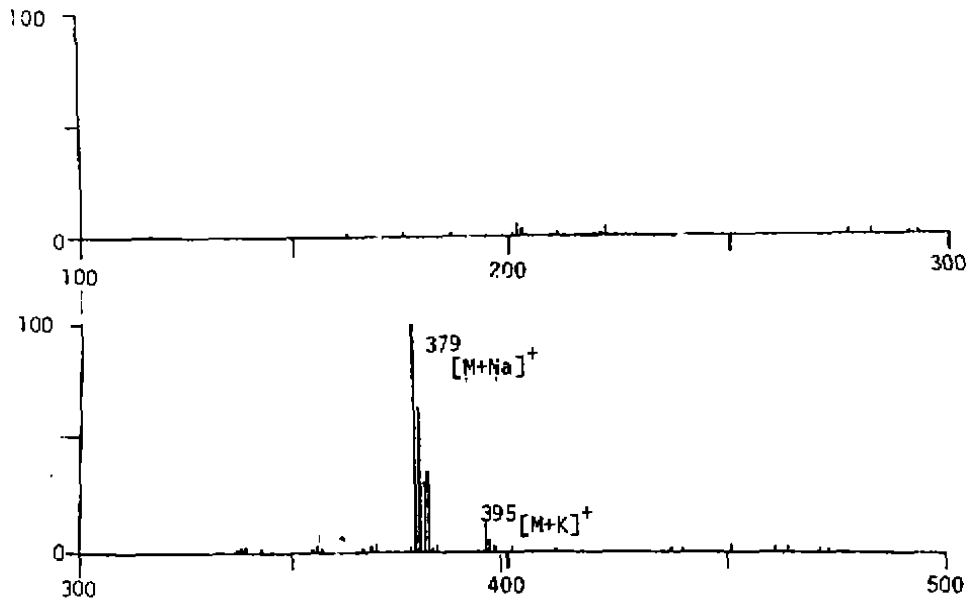
图 8 龙胆苦甙(13)的 FD-MS 谱图
