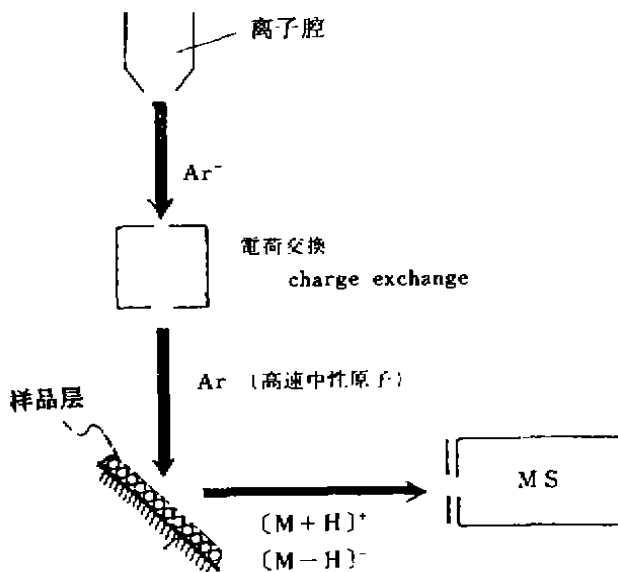
图2 FAB MS的原理
