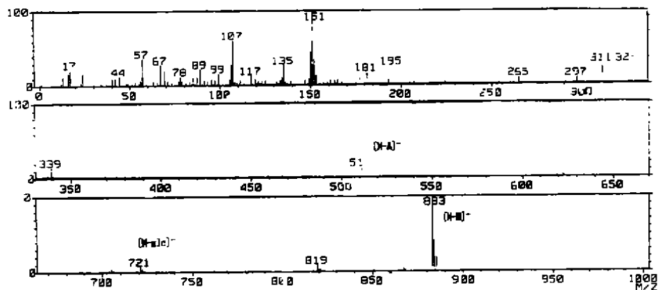
图 6 乌奴龙胆甙 C(23)的负离子 FAB-MS 谱图
