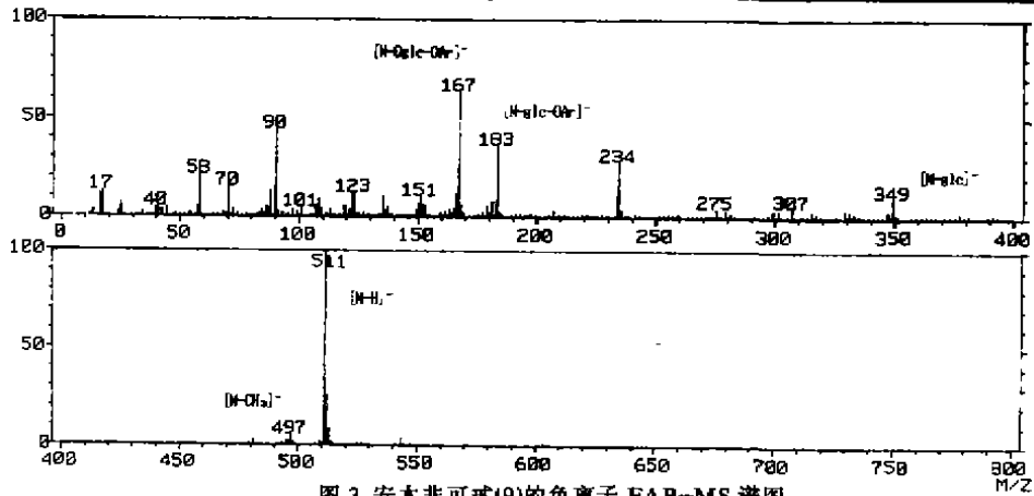
图3 安木非可甙(9)的负离子 FAB-MS 谱图
