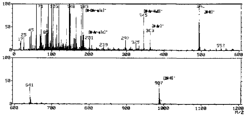
图5 哈巴俄甙(5)的负离子 FAB-MS 谱图
