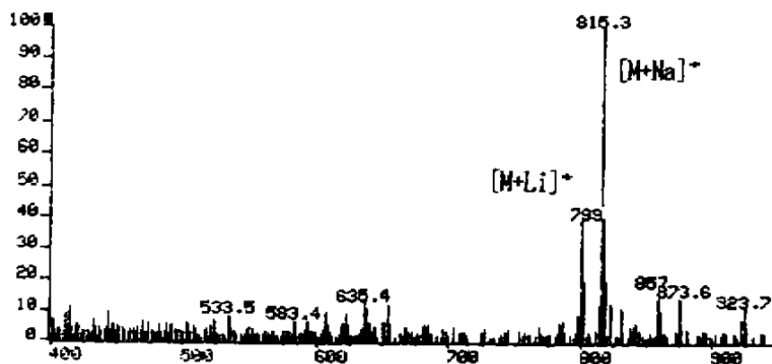
图 7 大花双参甙 A(22)的正离子 FAB-MS 谱图
